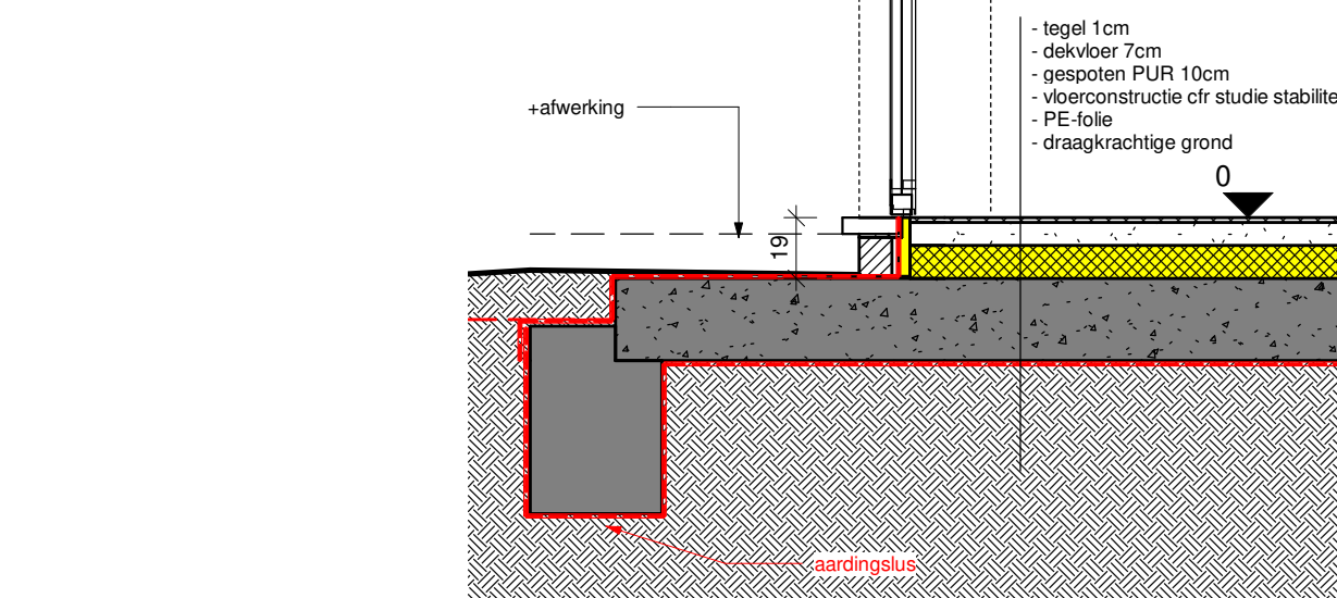
13 det 4 - inkom 1 : 25
