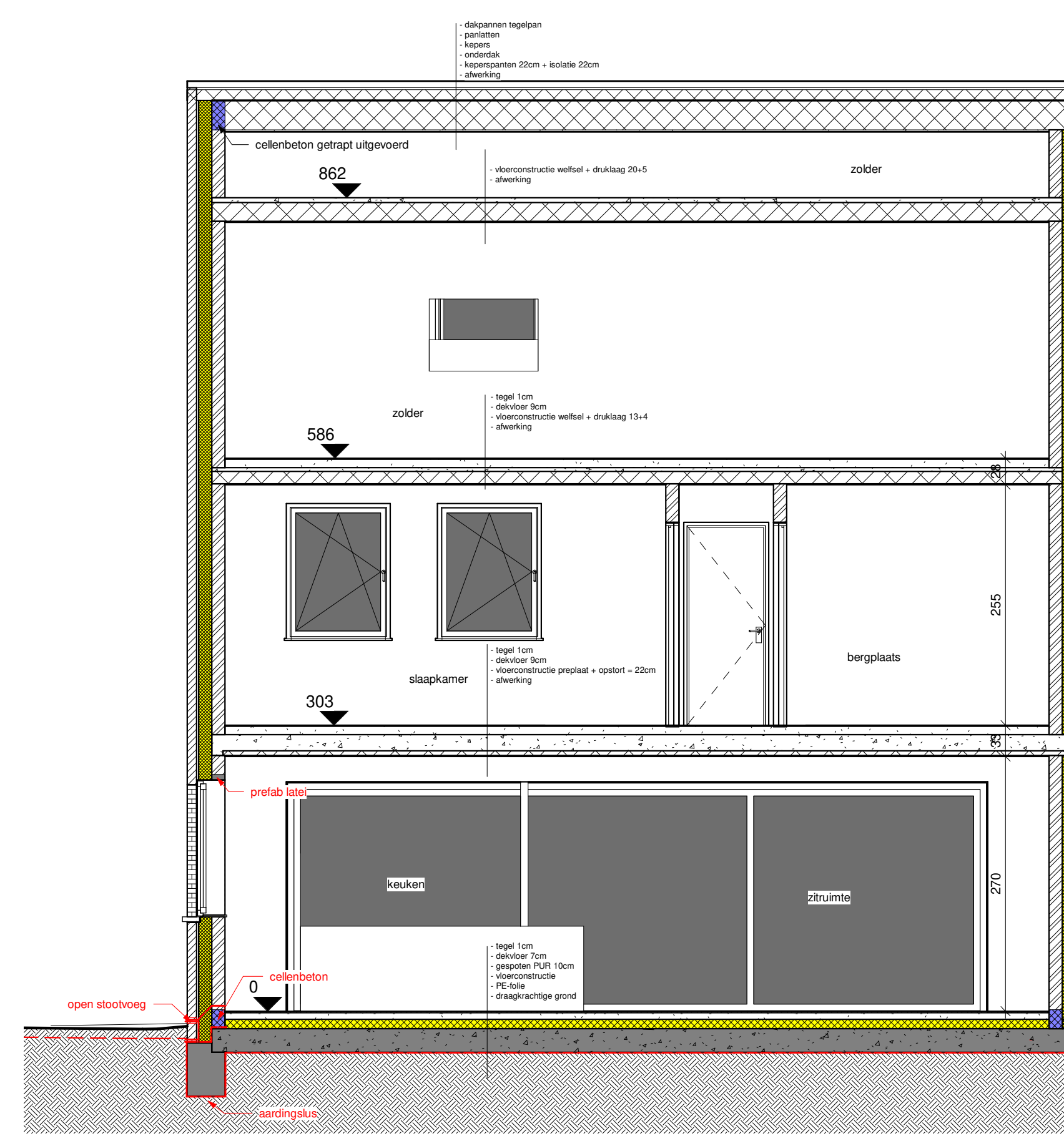
SNEDE 3 NT SCHAAL 1/50
