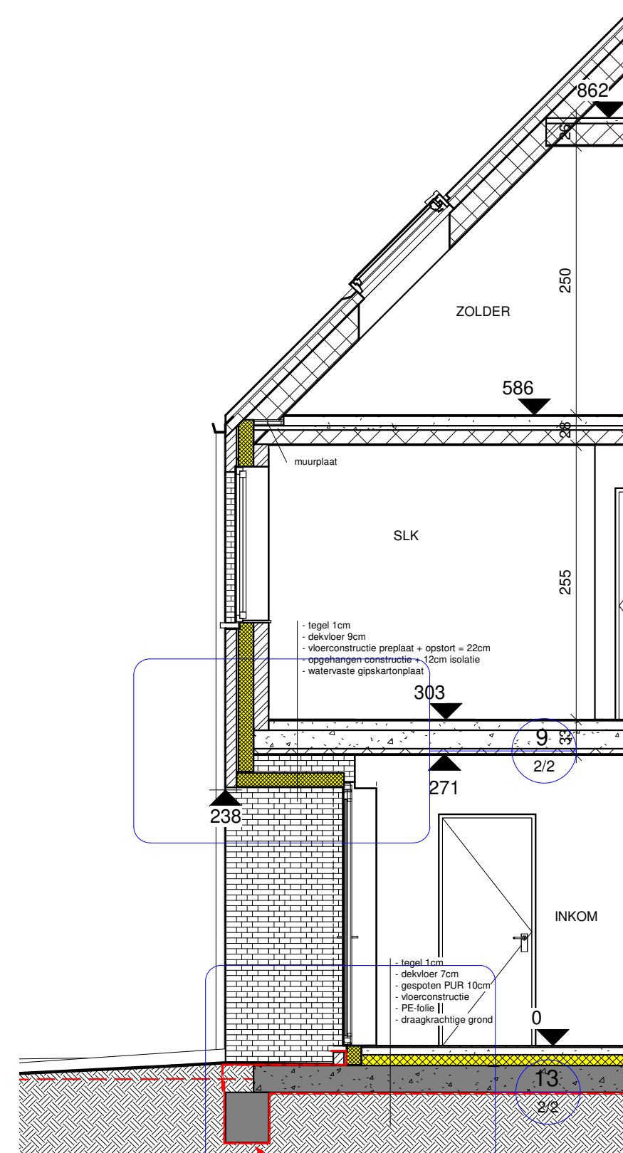
SNEDE 2 NT SCHAAL 1/50
