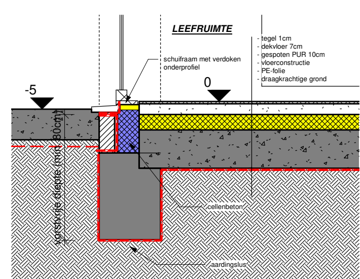
8 det 2 - onder schuifraam 1 : 25
