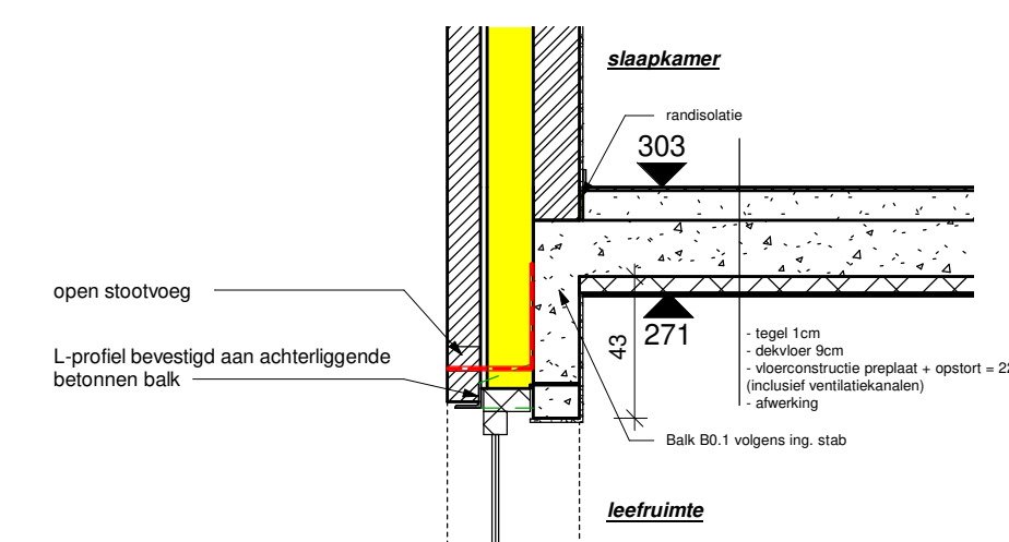
7 det 1 - boven schuifraam 1 : 25
