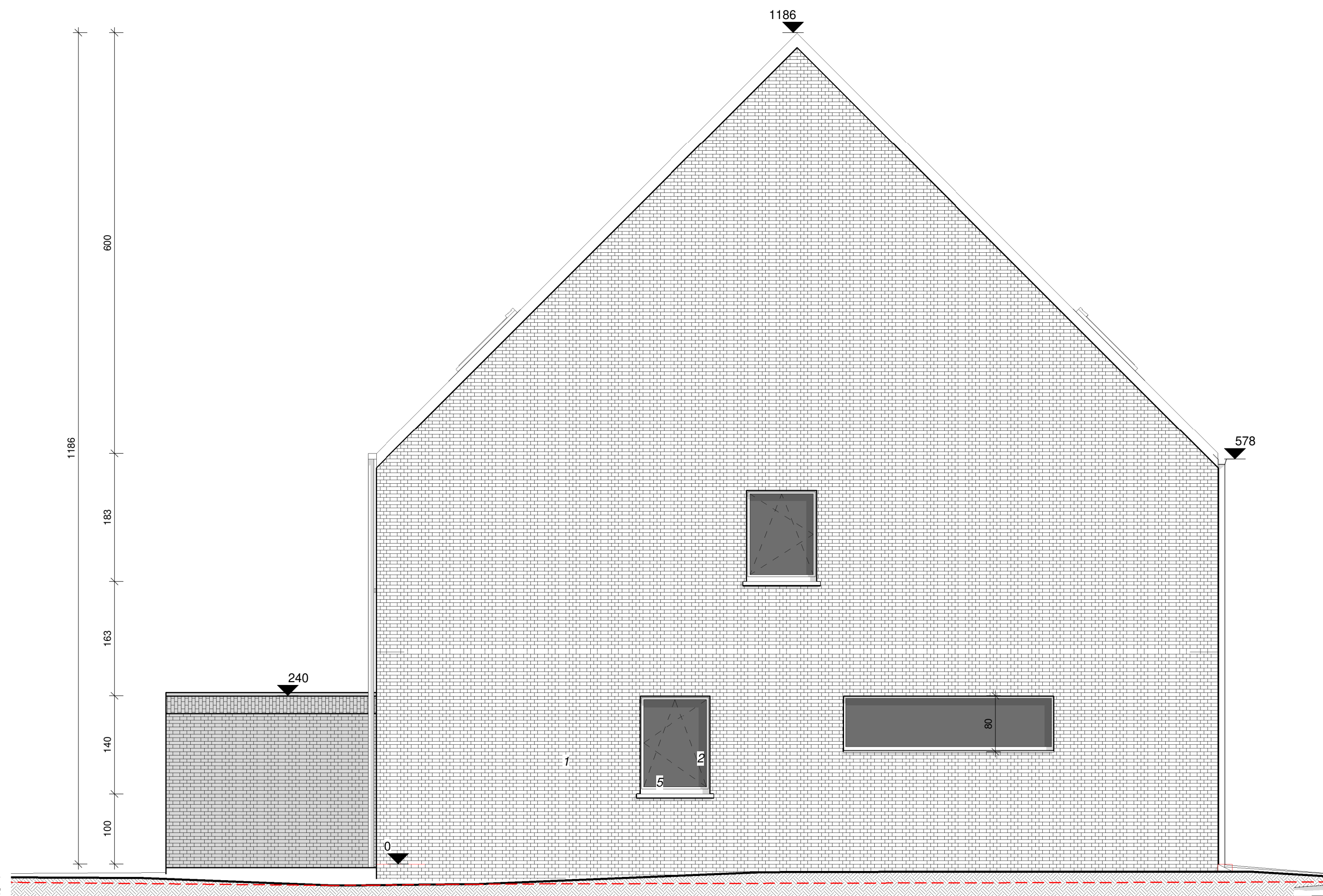
LINKERGEVEL NT SCHAAL 1/50
