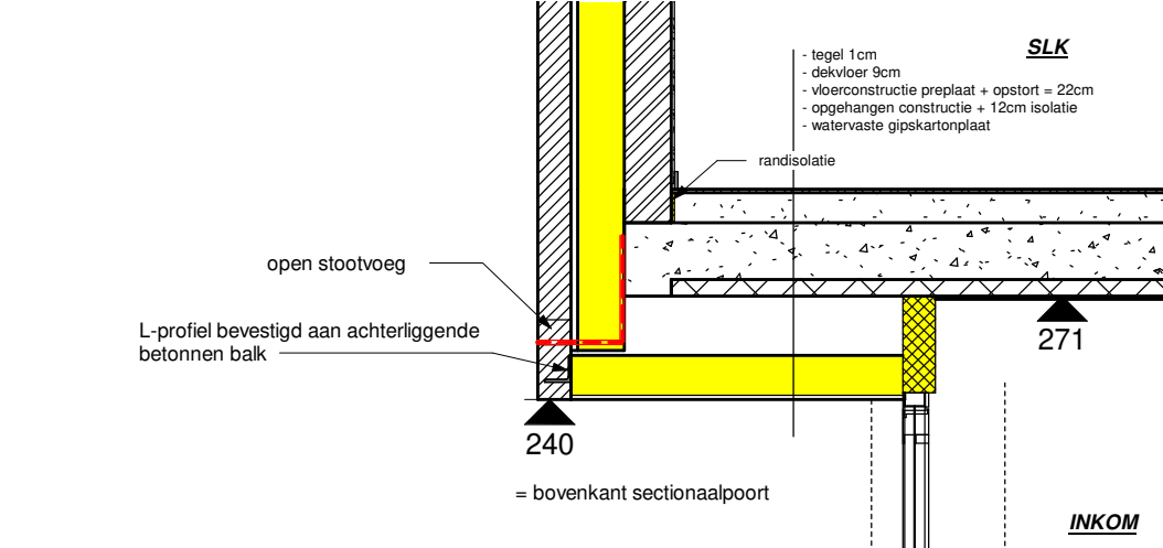
9 det 3 - boven inkom 1 : 25
